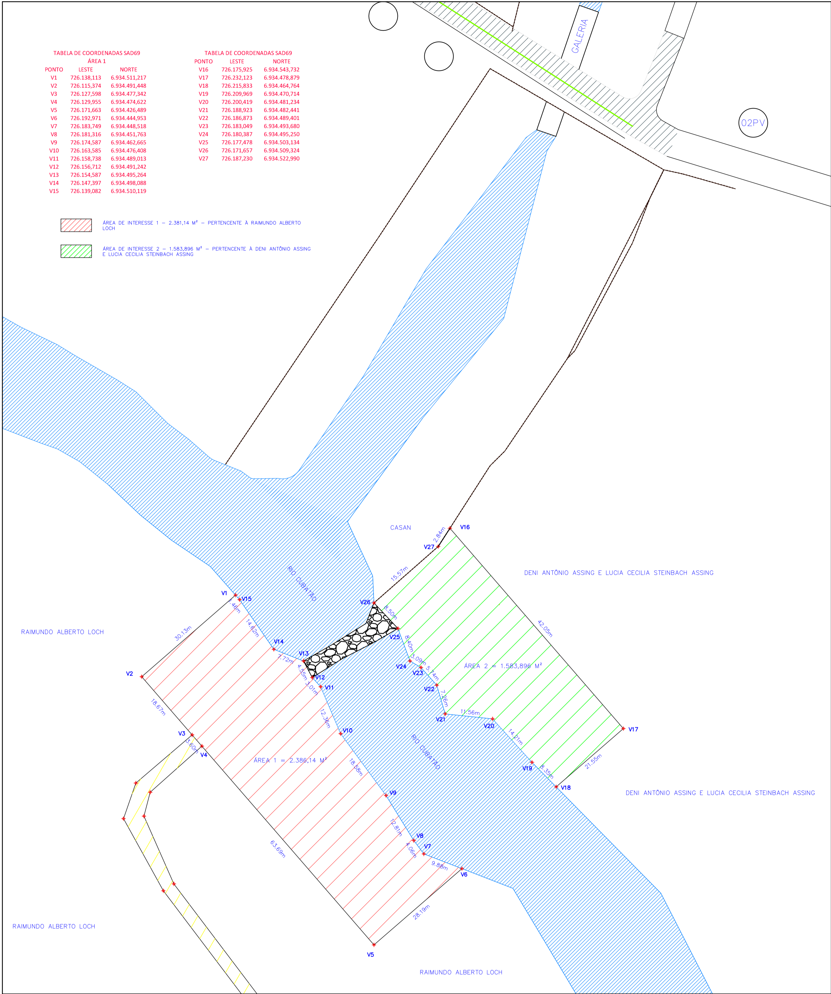
1 PLANTA DE LOCAÇÃO ESCALA 1:500
